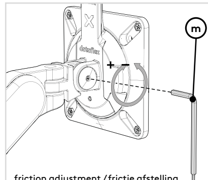
friction adjustment / frictie afstelling Friktionseinstellung / réglage du frottement regolazione dell'attrito / ajuste de fricción
