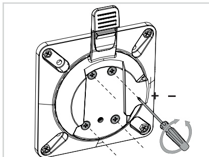
friction adjustment / frictie afstelling Friktionseinstellung / réglage du frottement regolazione dell'attrito / ajuste de fricción
